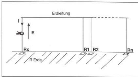
Schaltbild der Prüfung mit Erdungsprüfzange
