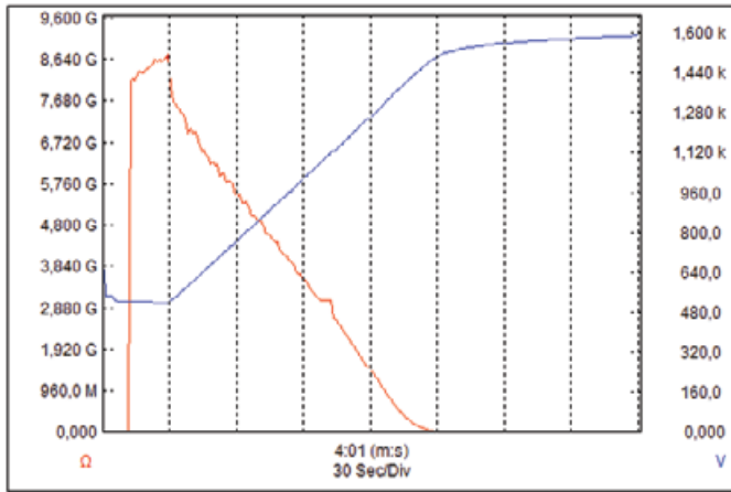
MÓDULO MEG Trazado gráfico de las pruebas V(t), R(t) en resistencia de aislamiento no lineal
