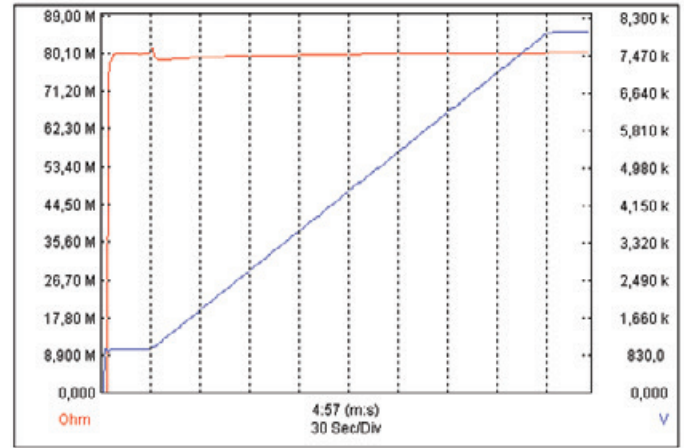
MÓDULO MEG Trazado gráfico de las pruebas V(t), R(t) en resistencia de aislamiento fija lineal (protector de sobretensión)
