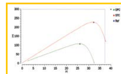
CURVA I-V
